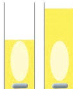
3. ábra. A fotokémiai reakció sebességének oldattér fogattól való függését szemléltető séma. A kuvettában található oldatot élénk-sárga szín jelöli, azt a részt pedig, ahol a fotométer fénye átmegy a mintán, halványsárga. A kevertetés fontos ezen méréseknél (lásd: mágneses keverőtest a kuvettákban)
