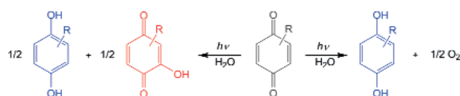
7. ábra. Kinonok vizes oldatában végbemenő fotokémiai reakciók
